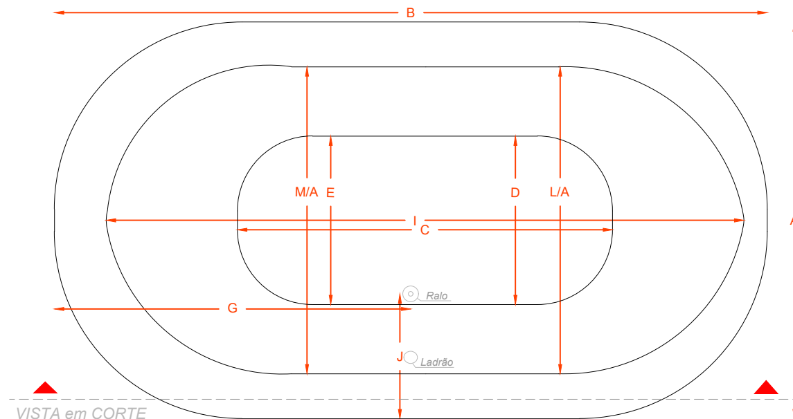
PLANTA BAIXA
